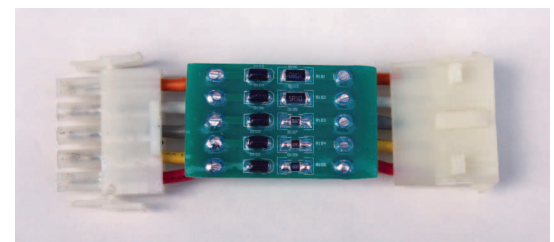
Image 5 : Carte de circuit imprimé du X-13
