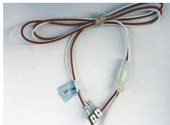
Imagen 7: arnés de cables de ajuste automático
