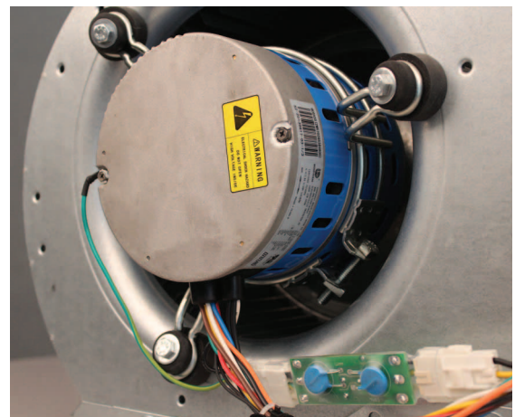
Image 1 : Orientation du moteur
