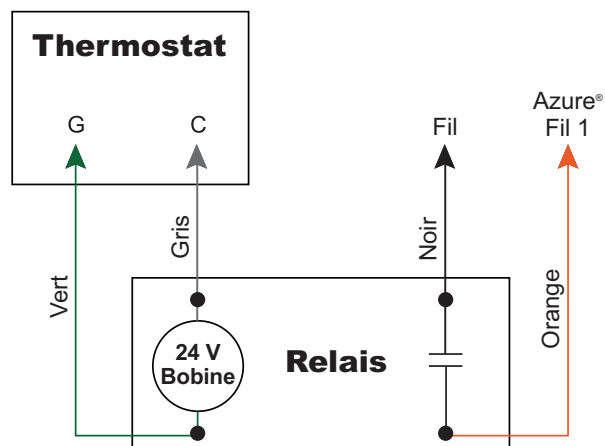
Diagramme de câblage C : Ensemble de ventilation constante
