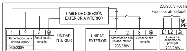
Diagrama de conexión (18K/24K)
