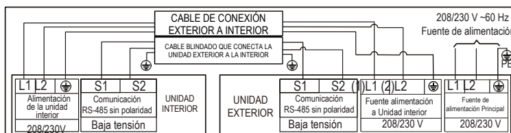
Diagrama de conexión (36K/48K/60K)
