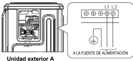
Unidad exterior A
